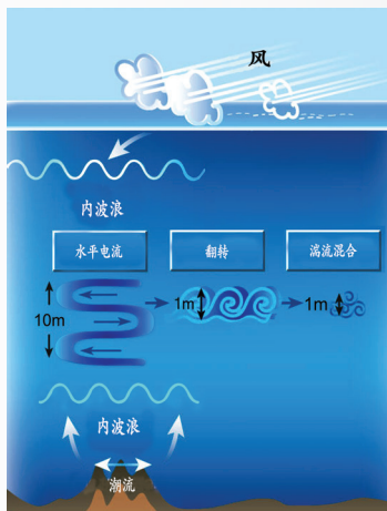
两层不同密度的水之间界面的内波。
